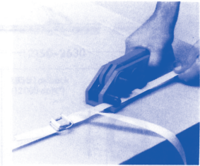
Spannapparat hinter der Schnalle plazieren Placer le tendeur derrière la boucle
