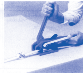
Band mit dem Hebel spannen Tirer sur la sangle et tendre à l'aide de la poignée
